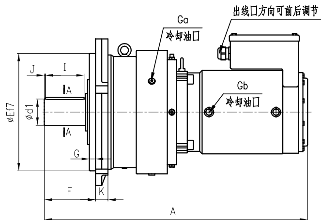
IEM1-***-01系列标准平键安装连接尺寸图
