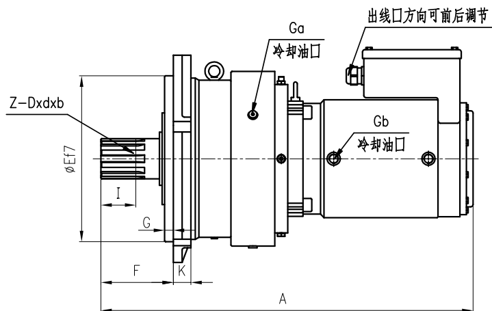
IEM1-***-01系列标准矩形外花键安装连接尺寸图
